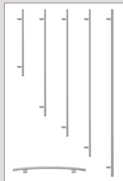
Maniglione (v.l.n.r.) 14032 (SG 403, 800 mm), 15096 (SG 405, 1200 mm), 15097 (SG 406, 1400 mm), 15098 (SG 407, 1600 mm), 14160 (SG 416, 600 mm), 155xx (Ø 40 mm) inox satinato, montaggio diretto, Modell A 12422 e A 12940 Maniglione 14030 (SG 403, 800 mm) montaggio inclinato
